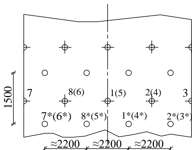
Развертка А-А
